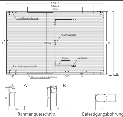
Rahmenquerschnitt
