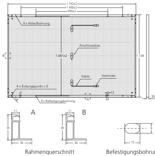
Rahmenquerschnitt
